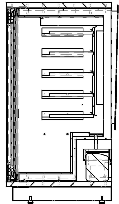
SEZIONE A-A
