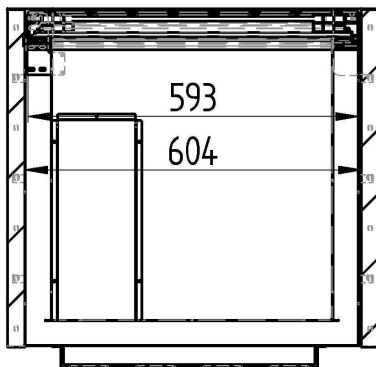
SEZIONE B-B
